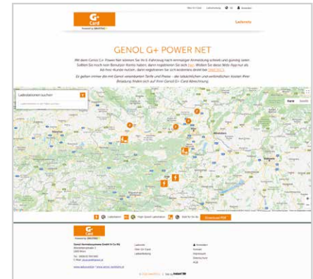
GENOL Web-App
